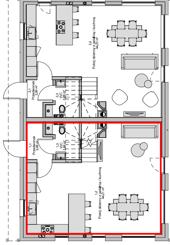
Budynek 1.1 - parter
